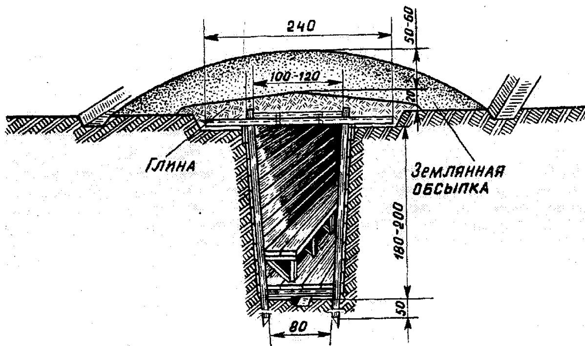
Рисунок 2.2 – Перекрытая щель (размеры даны в сантиметрах) Средства индивидуальной защиты
