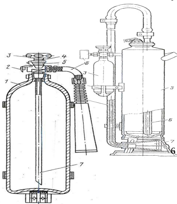
Рисунок 4 - Огнетушитель порошковый ОП – 10
