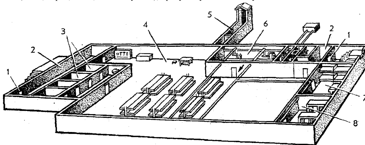
Рисунок 2.1 – План убежища
