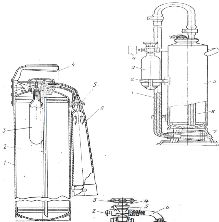
Рисунок 3- Углекислотный огнетушитель ОУ– 5
