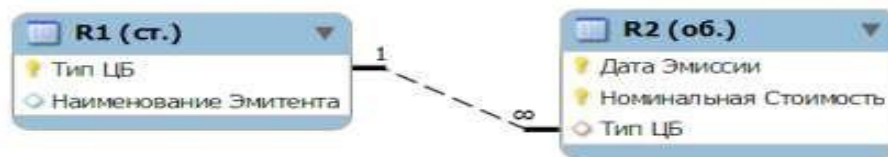
Рисунок 2.1. Схема «Таблица – связь»
