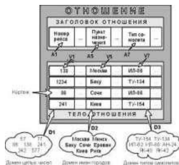
Рисунок 1.2. Отношение с математической точки зрения
