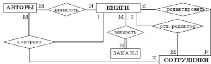
Рисунок 2. ER–диаграмма издательской компании
