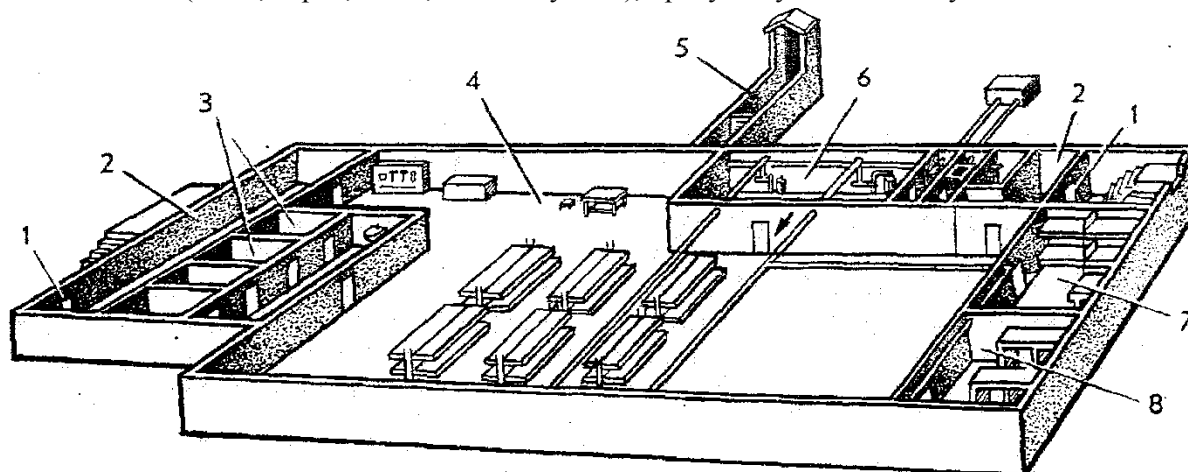
Рисунок 2.1 – План убежища
