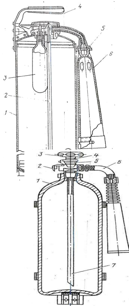
Рисунок 4 - Огнетушитель порошковый ОП – 10
